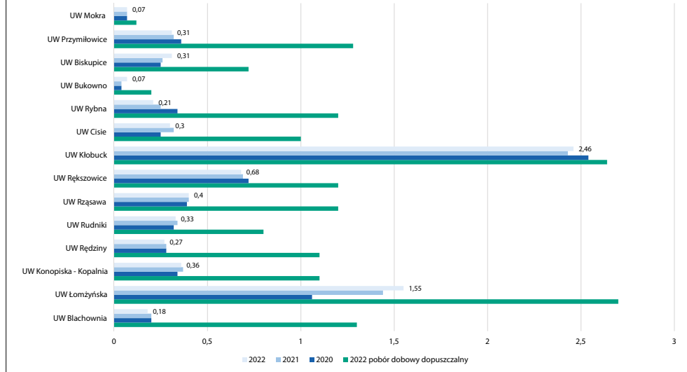
Pomocnicze ujęcia wody. Średniodobowa produkcja wody w latach 2020 - 2022 [tys. m 3 /dobę]
