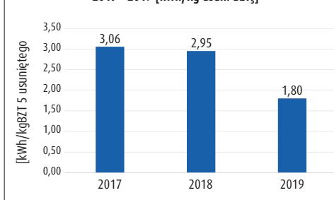
Zużycie energii elektrycznej na usunięcie 1 kg zanieczyszczeń (BZT 5 ) w oczyszczalni ścieków w Kolonii Pocznej w latach 2017 - 2019 [kWh/kg usun. BZT 5 ]
