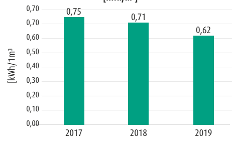
Zużycie energii elektrycznej na ujęcie i wtłoczenie wody z UW w Łobodnie do sieci wodociągowej w latach 2017 - 2019 [kWh/m 3 ]
