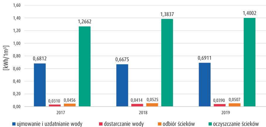
Jednostkowe zużycie energii elektrycznej na procesy: ujmowania i uzdatniania wody, dostarczenia wody, odbioru i oczyszczenia ścieków w latach 2017 - 2019 [ kWh/1m 3 ]
