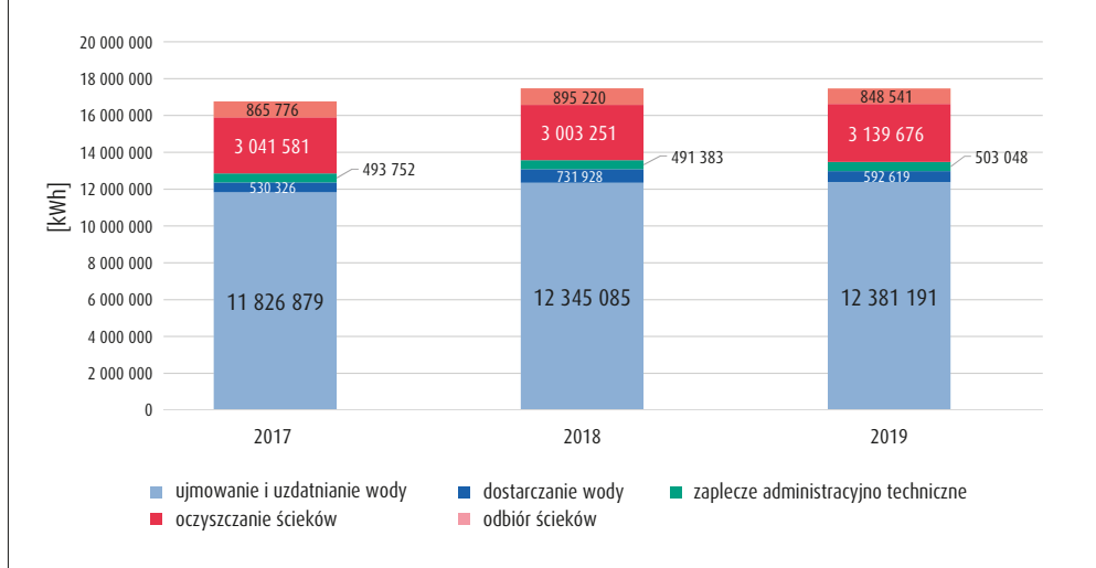
Zużycie energii elektrycznej na procesy: ujmowania i uzdatniania wody, dostarczenia wody oraz odbioru i oczyszczania ścieków w latach 2017 - 2019 [ kWh/rok]
