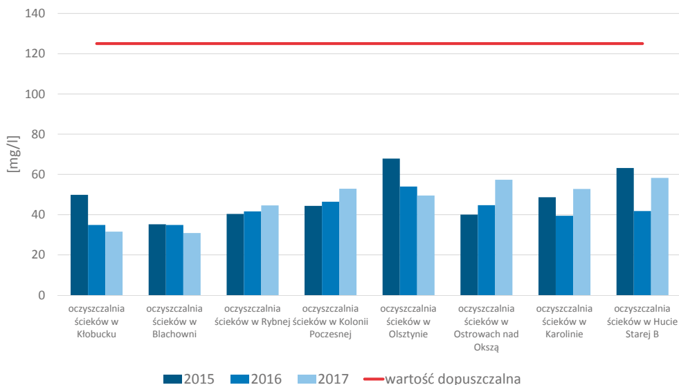
WYKRES 6. ŚREDNIOROCZNE STĘŻENIA WSKAŹNIKA CHZT W ŚCIEKACH OCZYSZCZONYCH ODPROWADZANYCH DO ODBIORNIKA W LATACH 2015 - 2017
