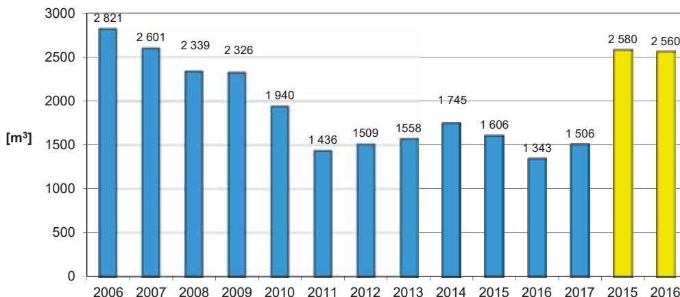
WYKRES 2. STRATY WODY W SIECI W LATACH 2006-2017
