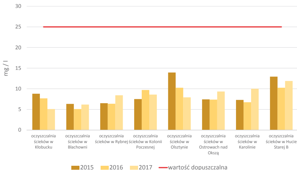
WYKRES 5. ŚREDNIOROCZNE STĘŻENIA WSKAŹNIKA BZT5 W ŚCIEKACH OCZYSZCZONYCH ODPROWADZANYCH DO ODBIORNIKA W LATACH 2015 - 2017
