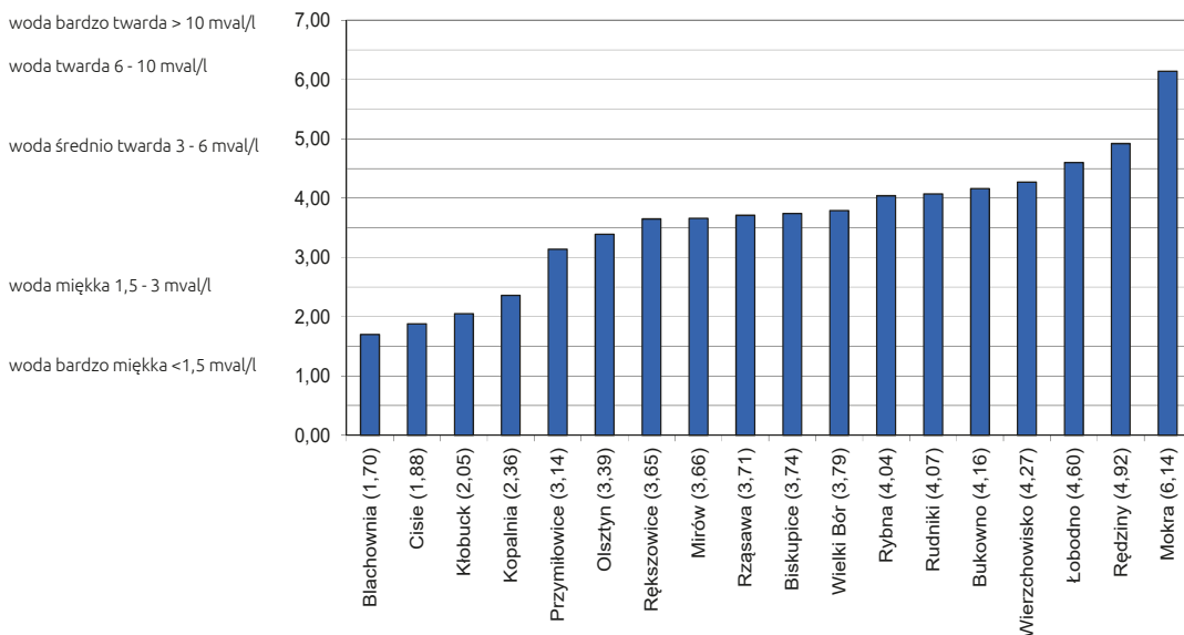
WYKRES 3. ŚREDNIE WARTOŚCI TWARDOŚCI WODY PODAWANEJ DO SIĘCI Z POSZCZEGÓLNYCH UJĘĆ [mval/l]
