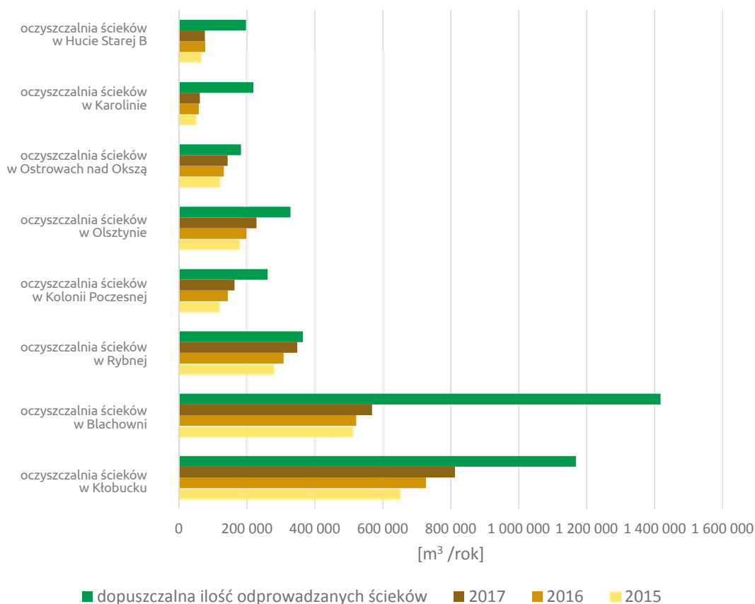
WYKRES 8. ILOŚĆ ODPROWADZONYCH ŚCIEKÓW OCZYSZCZONYCH Z POSZCZEGÓLNYCH OCZYSZCZALNI W LATACH 2015 - 2017 [m 3 /rok]
