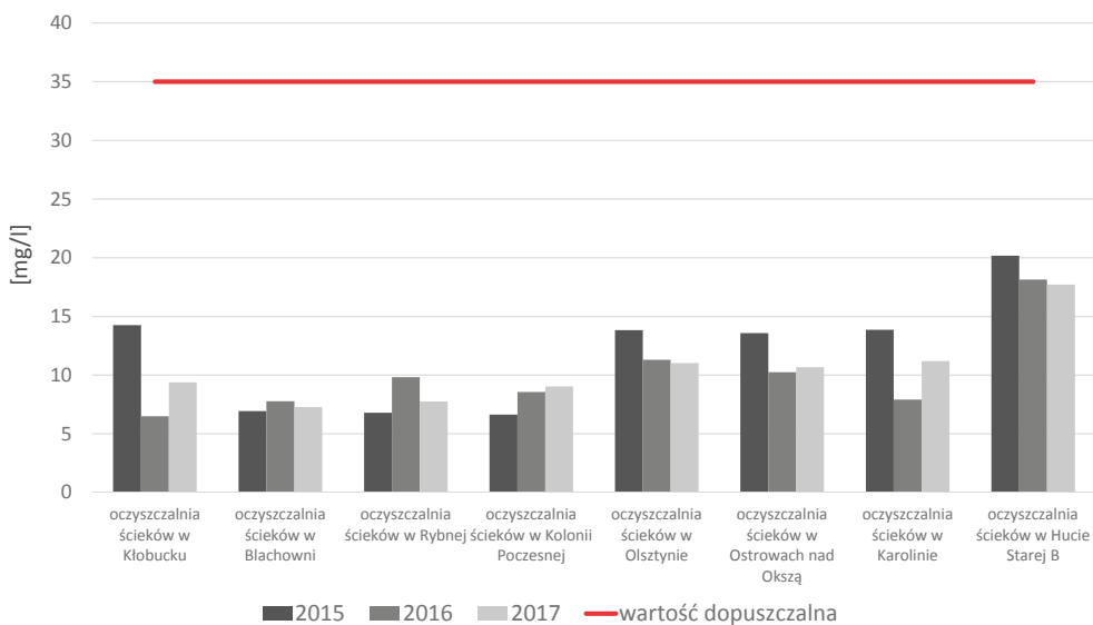
WYKRES 7. ŚREDNIOROCZNE STĘŻENIA WSKAŹNIKA ZAWIESINY W ŚCIEKACH OCZYSZCZONYCH ODPROWADZANYCH DO ODBIORNIKA W LATACH 2015 - 2017
