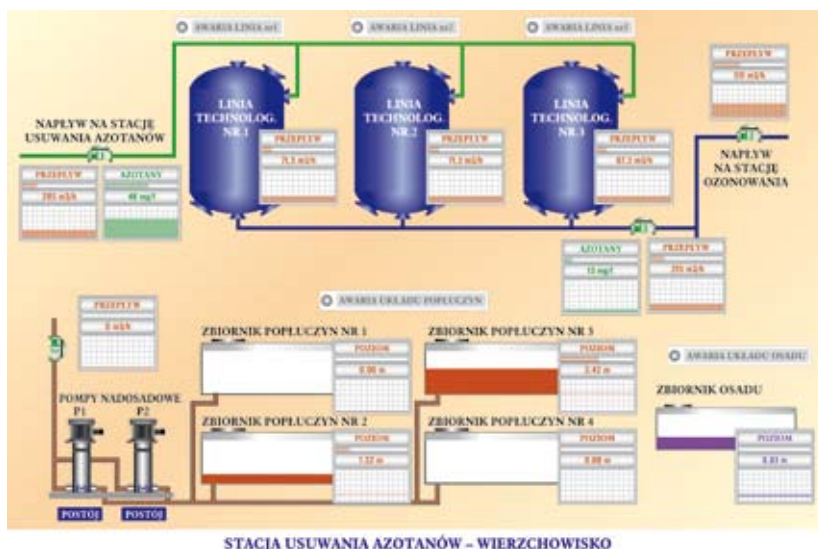
STACJA USUWANIA AZOTANÓW - WIERZCHOWISKO
