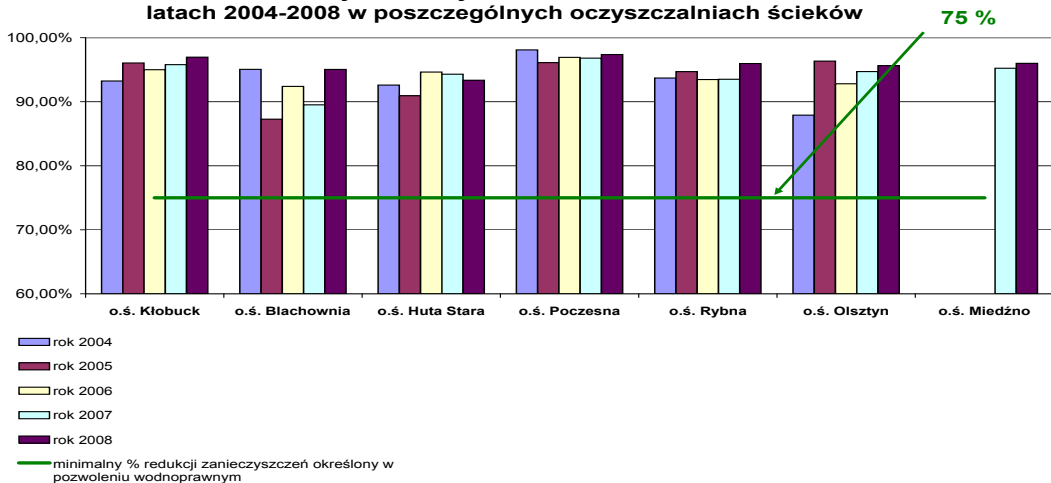
Średnioroczna redukcja zanieczyszczeń mierzona wskaźnikiem zawiesiny w latach 2004-2008 w poszczególnych oczyszczalniach
