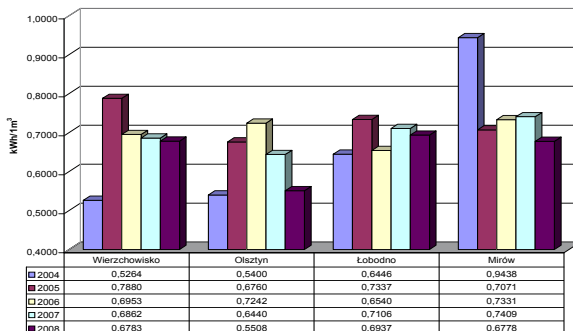
Zużycie energii elektrycznej na pobór i dezynfekcję 1 m³ wody w latach 2004-2008
