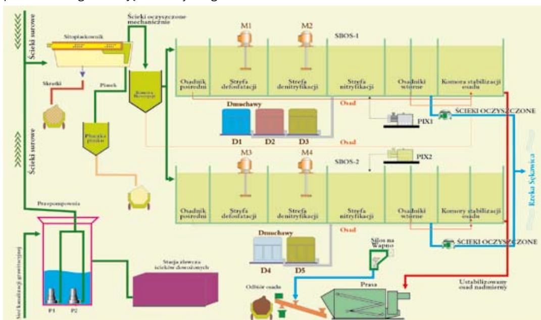
SCHEMAT TECHNOLOGICZNY OCZYSZCZALNI SUPERBOS W RYBNEJ
